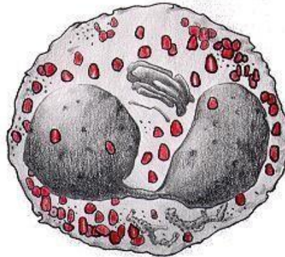
Fig. 9 - Eosinophil
